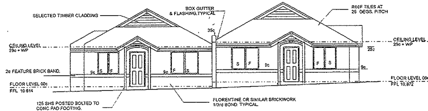
ELEVATION 9 1:100
