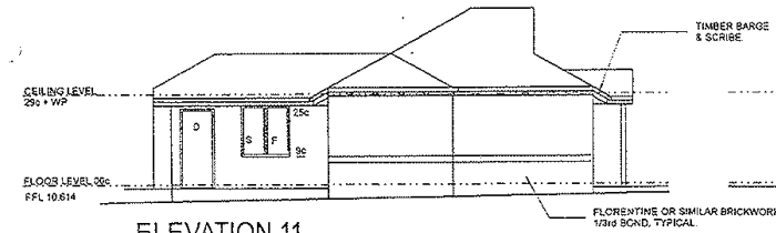
ELEVATION 11 1:100
