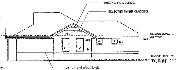
ELEVATION 12 1:100
