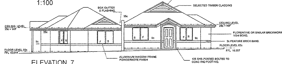
ELEVATION 7 1:100
