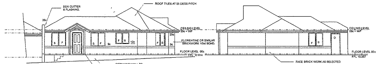
ELEVATION 5 1:100
