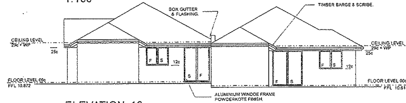
ELEVATION 10 1:100
